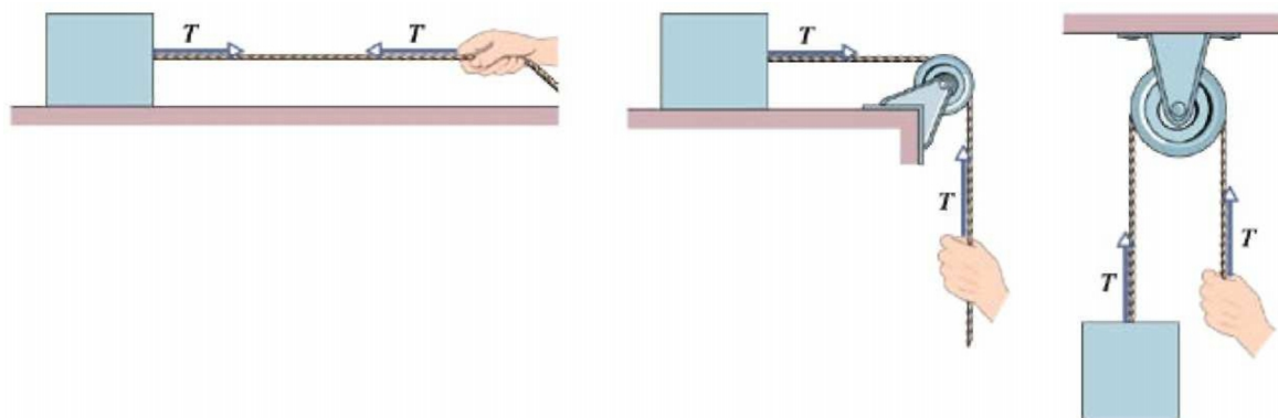
Figura 5.6: La corda è soggetta a tensione ed esercita una trazione sui corpi fissati ai due capi con una forza T (sinistra). Lo stesso vale nel caso in cui la corda scorra intorno a una puleggia priva di massa e di attrito (centro e destra).
