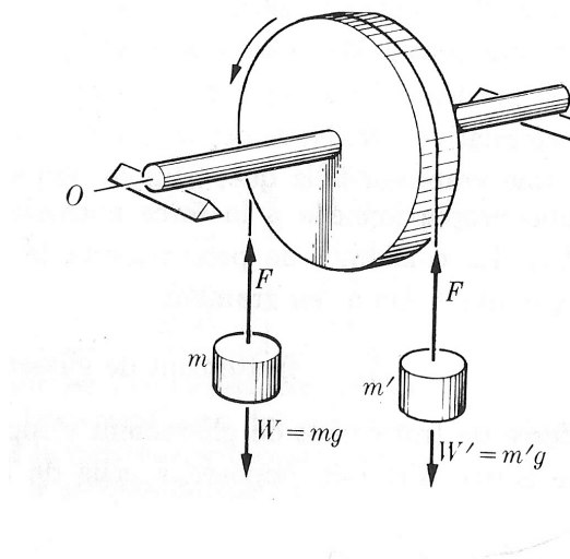
Figura 5.11: La macchina di Atwood
