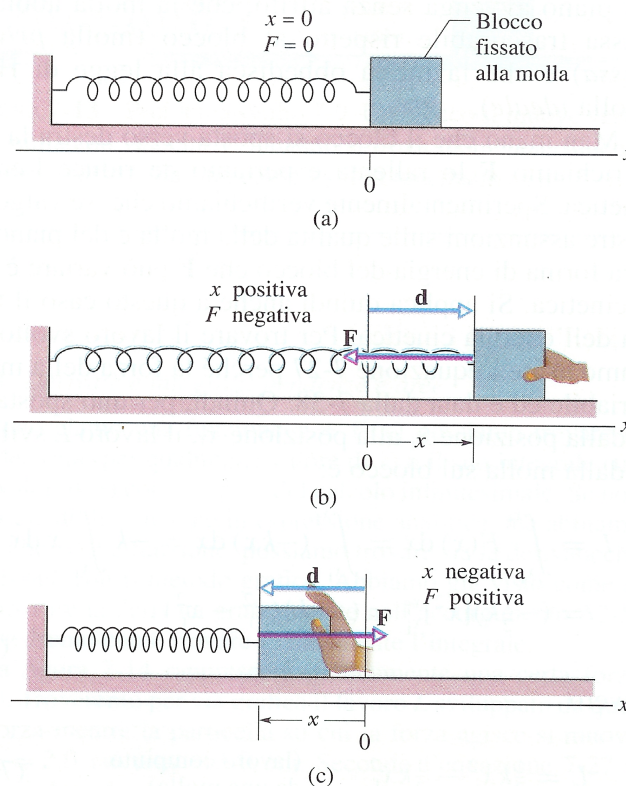
Figura 5.13: (a) molla a riposo (b) il corpo viene spostato di \vec{d} e la molla si allunga di x (c) la molla viene schiacciata di una lunghezza x
