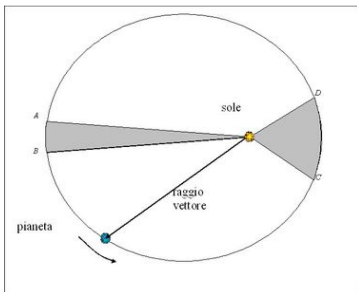
Figura 7.2: La legge delle aree
