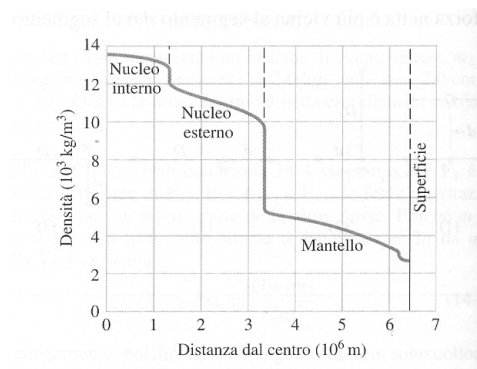
Figura 7.7: Densità della Terra in funzione della distanza dal centro.
