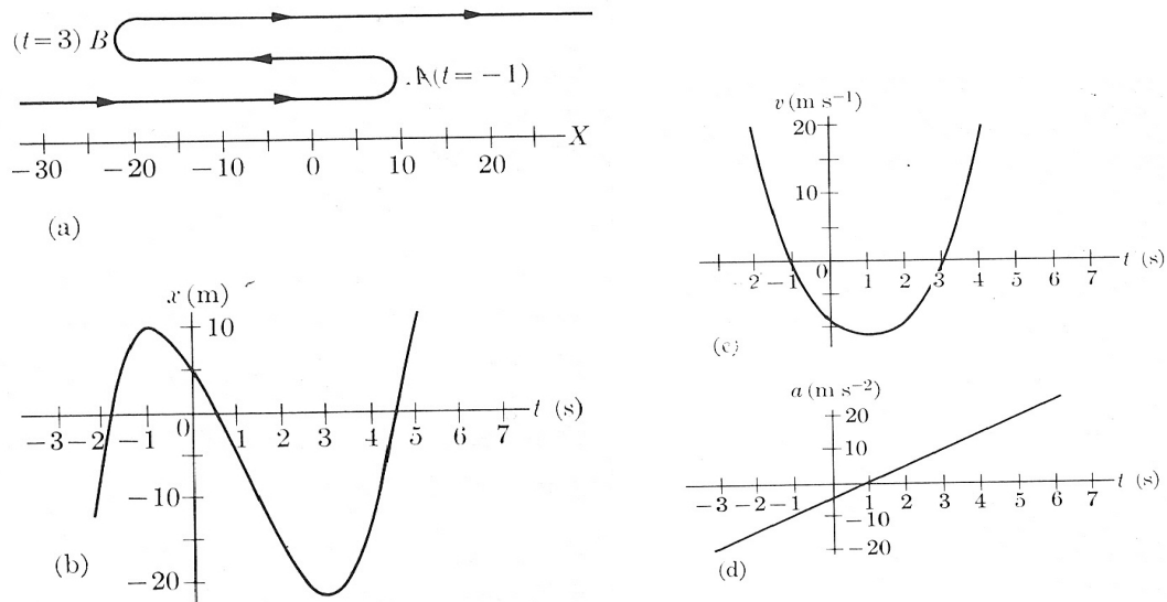
Figura 3.14: La traiettoria (a) e i grafici x(t) , v(t) e a(t) (b,c,d) per il moto non m.u.a.
