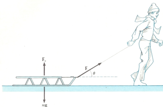
Figura 6.1: Un ragazzo che tira una slitta. Il lavoro compiuto durante uno spostamento \Delta x è pari a F\Delta x \cos \theta
