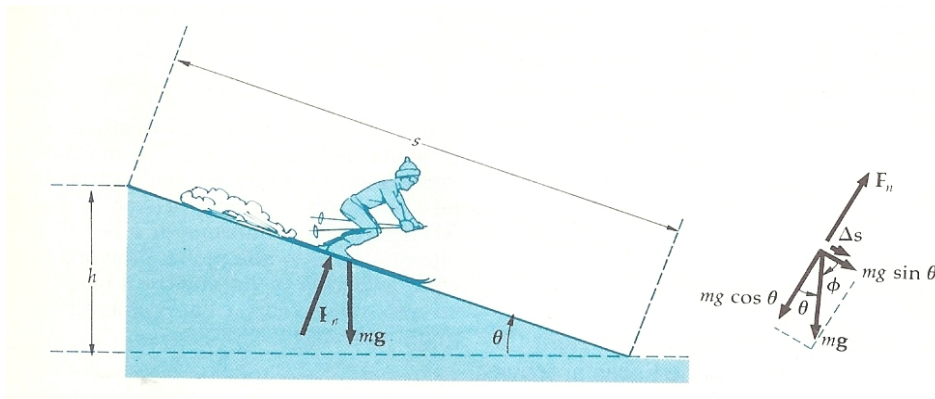
Figura 6.4: Lavoro della forza peso su un pendio a inclinazione costante
