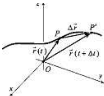
Figura 3.2: Vettore spostamento definito da due istanti successivi.
