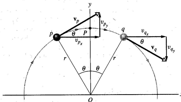
Figura 4.2: Una particella si muove di moto circolare uniforme a velocità scalare v costante su un cerchio di raggio r . Sono indicate le sue velocità \vec{v}_p e \vec{v}_q e le rispettive componenti, nei punti p e q equidistanti dall'asse y .
