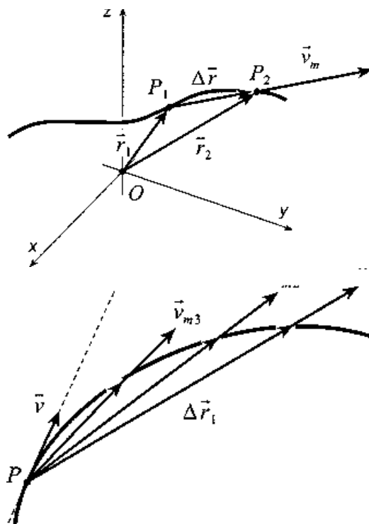
Figura 4.1: La velocità media e quella istantanea
