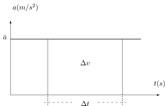
Figura 3.10: \Delta v quando a è costante
