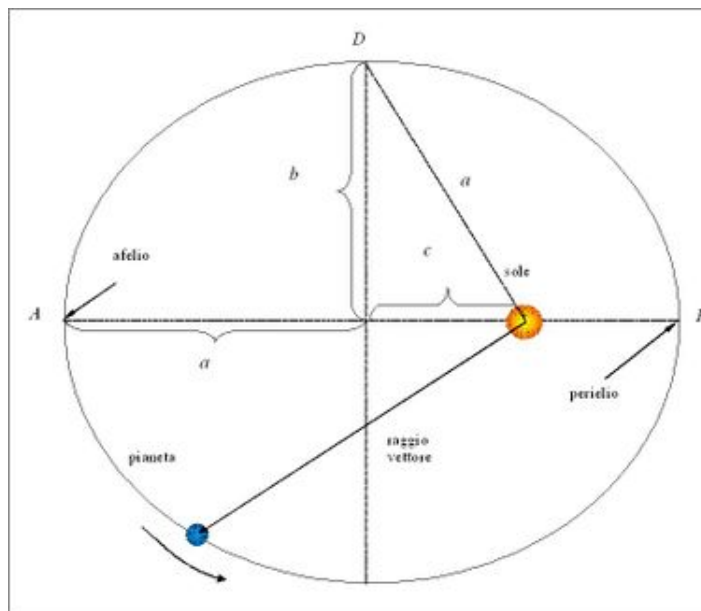
Figura 7.1: Un pianeta di massa m percorre un'orbita ellittica attorno al Sole.
