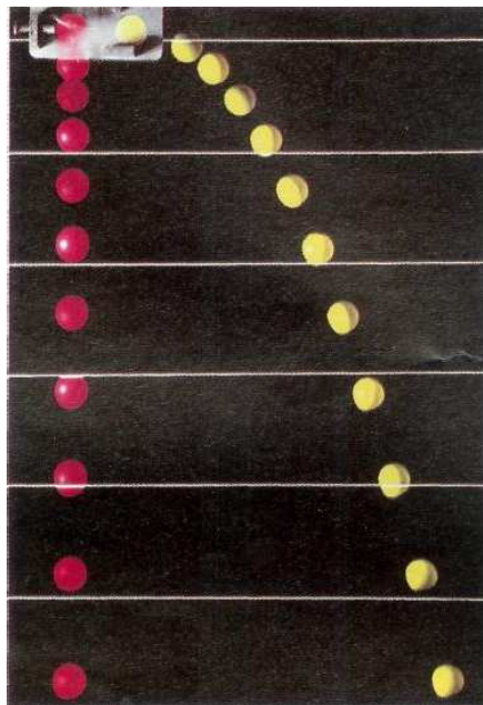
Figura 4.6: Una palla è lasciata cadere da ferma nello stesso istante in cui un'altra è sparata orizzontalmente verso destra. I loro moti verticali sono identici.
