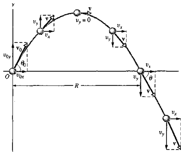
Figura 4.10: Traiettoria di un proiettile. Sono indicate, con le rispettive componenti, la velocità iniziale e le velocità in diversi punti lungo la traiettoria.
