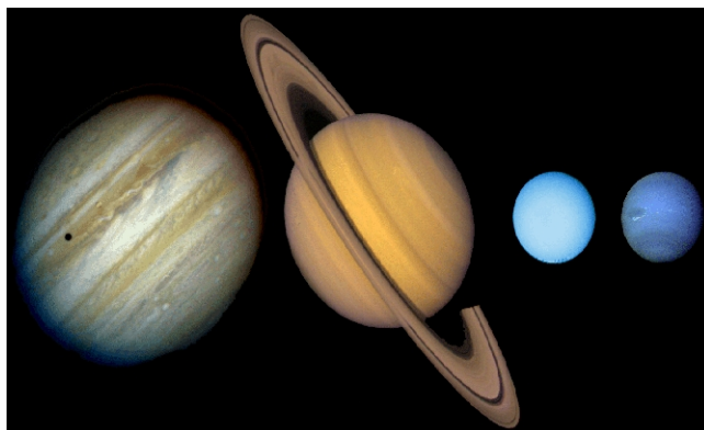
Figura 7.5: I pianeti gioviani. Le dimensioni sono in scala.
