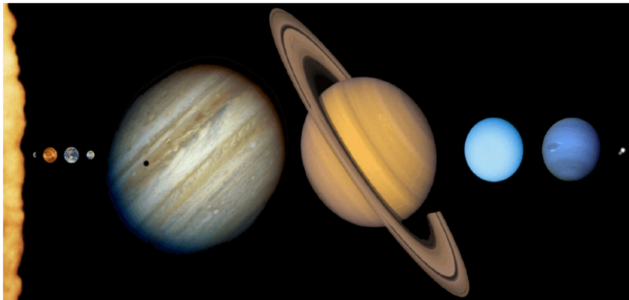
Figura 7.3: Il Sole e i pianeti approssimativamente nella scala reale.
