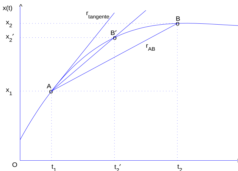
Figura 3.5: La velocità istantanea è la pendenza della retta tangente al grafico x(t)
