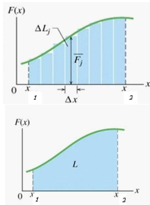
Figura 6.3: Lavoro di una forza variabile
