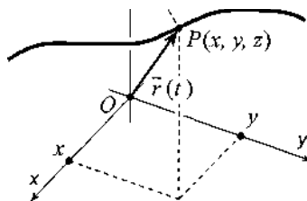
Figura 3.1: Traiettorie descritte dal vettore posizione \vec{r}(t) .
