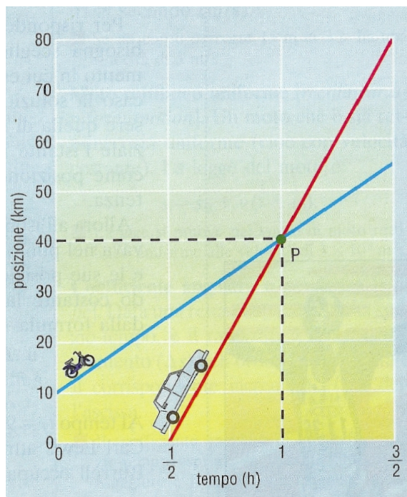
Figura 3.12: Nella figura sopra è rappresentata la soluzione grafica. L'auto raggiunge il motorino un'ora dopo la prima partenza, a una distanza di 40 km. Da notare che in questo caso è possibile utilizzare le unità di misura non SI dato che si tratta di uguaglianze.
