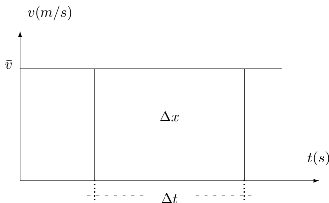
Figura 3.8: \Delta v quando a è costante
