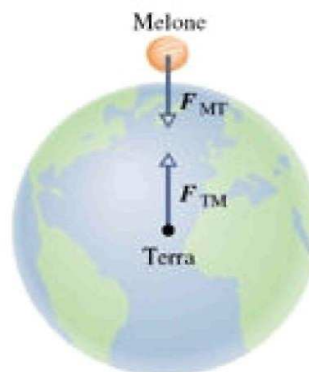
Figura 5.3: La forza esercitata dalla Terra sul melone è uguale a quella fatta dal melone sulla Terra
