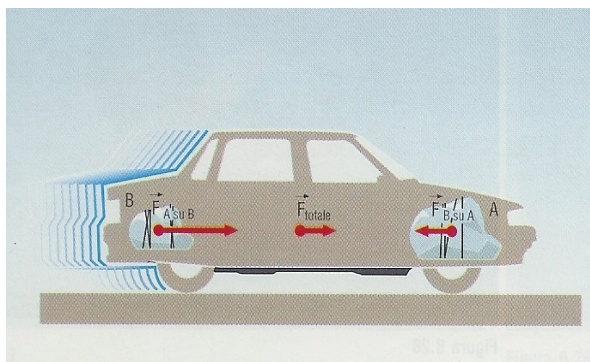
Figura 5.4: Se il terzo principio fosse falso, l'auto accelera senza carburante!
