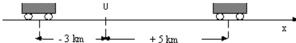
Figura 3.3: Due posizioni determinate su una asse che si estende all'infinito
