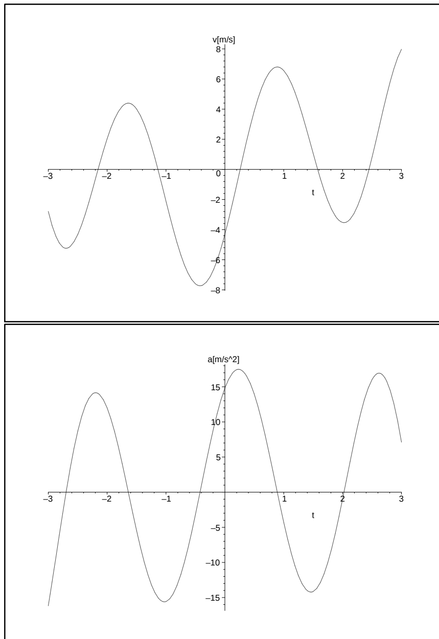
Figura 3.7: Il grafico v(t) e il grafico a(t) corrispondente
