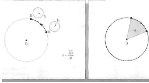
Figura 4.3: Velocità periferica e angolare
