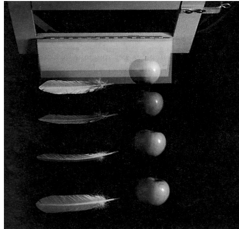
Figura 4.5: Una mela e una piuma in caduta libera nel vuoto
