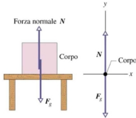
Figura 5.7: Il corpo appoggiato su un tavolo, è soggetto a una forza normale N perpendicolare al piano del tavolo. A destra il corrispondente diagramma delle forze.
