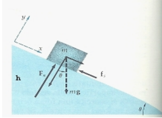
Figura 6.7: Un corpo scivola lungo un piano inclinato.
