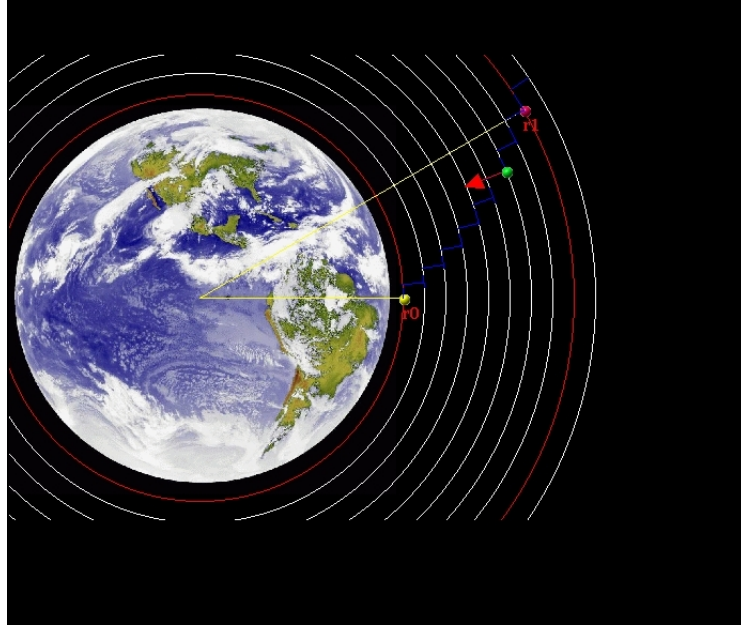
Figura 7.6: Spostamento di una massa m da un'orbita a un'altra.
