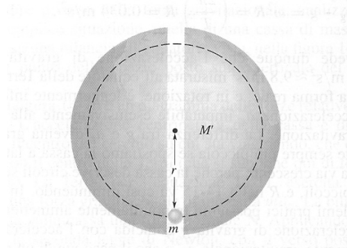
Figura 7.9: Una particella è lasciata cadere in una galleria scavata attraverso la Terra.
