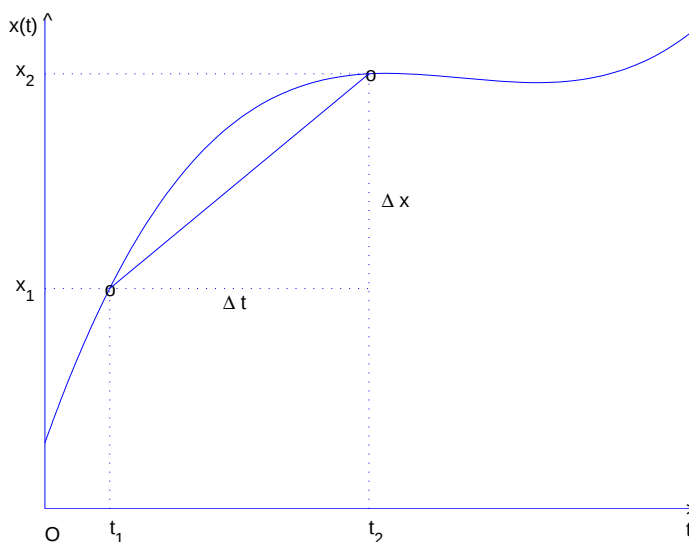
Figura 3.4: La velocità media è la pendenza della retta che congiunge i due punti sul grafico x(t) .
