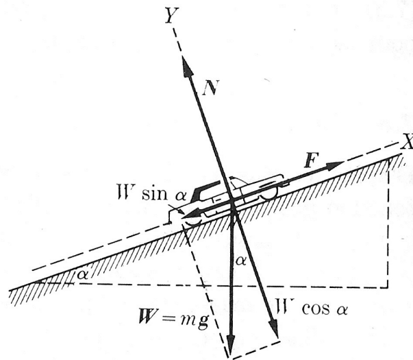
Figura 5.12: Auto in salita
