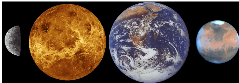
Figura 7.4: I pianeti tellurici. Le dimensioni sono in scala.
