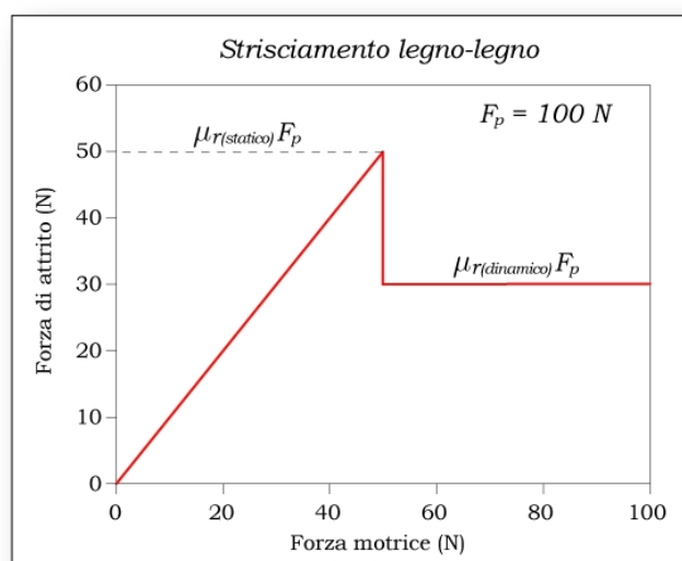
Figura 5.8: Grafico del valore della forza di attrito radente in funzione della forza applicata. Qui F_p = 100 N è la forza di contatto. Si noti il passaggio da attrito statico ad attrito dinamico, coincidente con l'inizio del moto del corpo.
