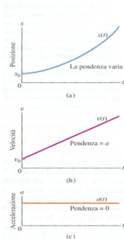
Figura 3.13: I tre grafici x(t) , v(t) , a(t) per il caso in cui a > 0
