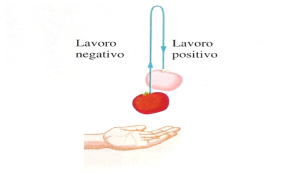
Figura 6.2: Un pomodoro lanciato in aria. Durante la salita il suo peso compie un lavoro negativo, durante la discesa il suo peso compie un lavoro positivo.
