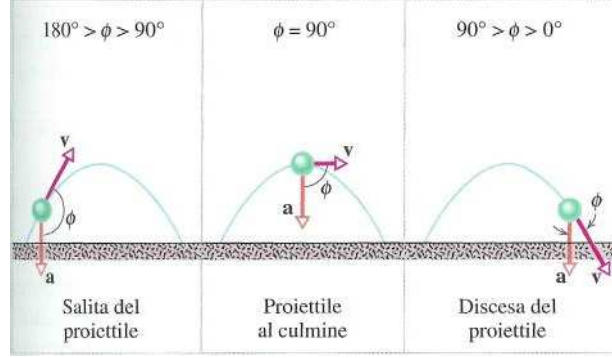
Figura 4.11: Vettori velocità e accelerazione di un proiettile in diversi istanti. Si noti che le direzioni dei due vettori non presentano alcuna relazione fissa.
