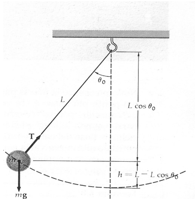
Figura 6.5: Il pendolo semplice
