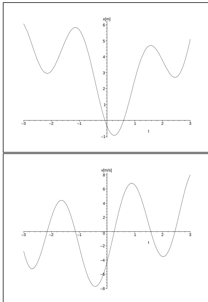
Figura 3.6: Il grafico x(t) e il grafico v(t) corrispondente
