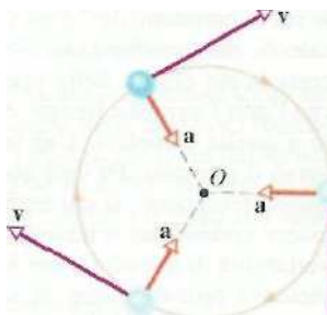
Figura 4.4: Vettori velocità e accelerazione per una particella in moto circolare uniforme.
