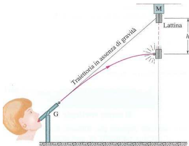
Figura 4.8: La pallina colpisce sempre la lattina. Entrambe cadono di un'uguale altezza h dal punto in cui si incontrerebbero se non esistesse l'accelerazione di gravità
