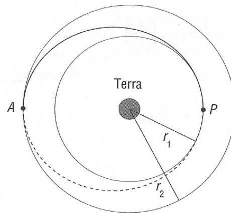
Figura 7.8: Orbita di trasferimento: sono indicati il perielio (P) e l'afelio (A).
