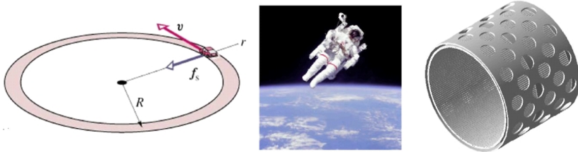
Figura 5.9: Esempi di forza centripeta
