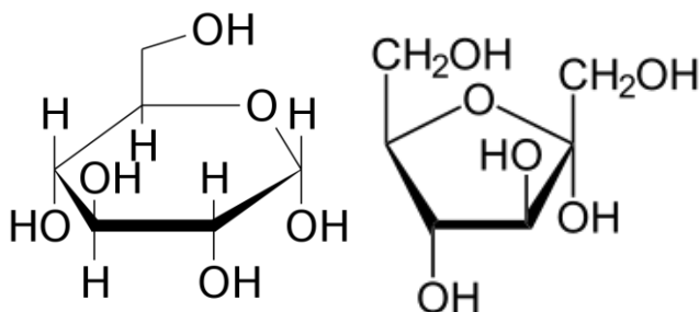
Struttura atomica di glucosio e fruttosio C_6H_{12}O_6
