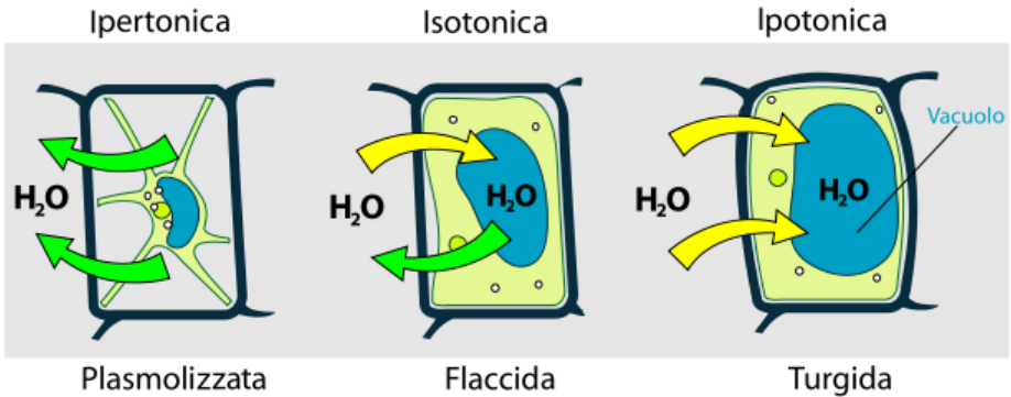
Effetto dell'osmosi nelle cellule vegetali
