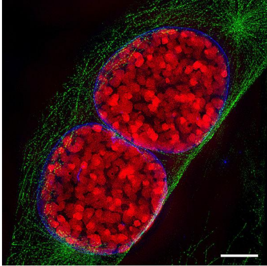
Due nuclei cellulari in profase. La barra della scala è lunga 5 \mu m.
